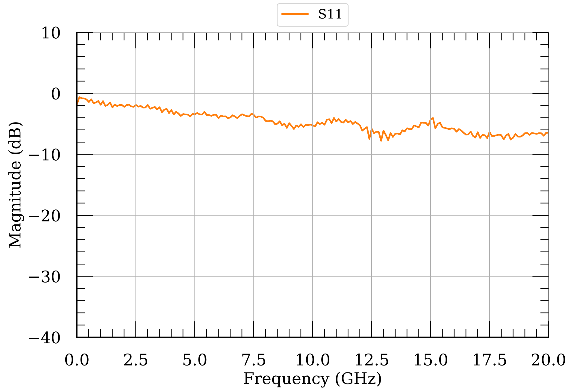
LNA S-params module094
